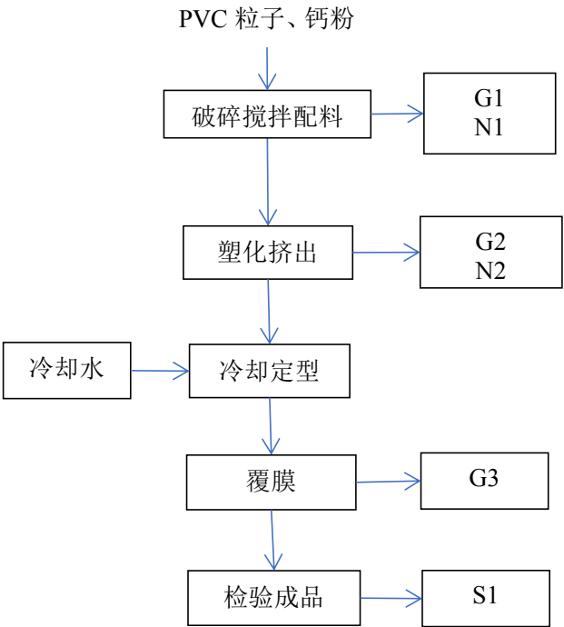
图 2-2 生产工艺流程图
